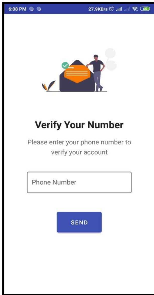
Fig.3.6.1 Login Page
